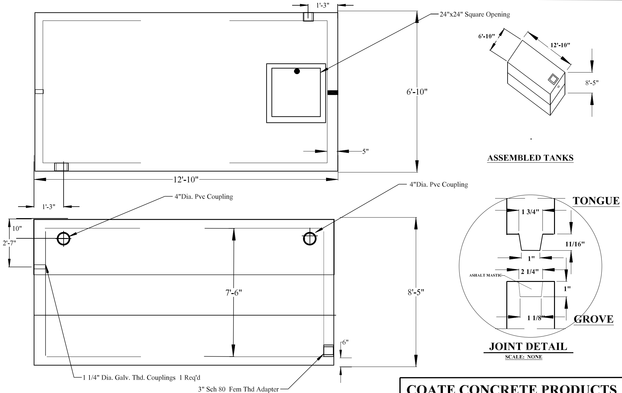
4000 Gallon Cistern
